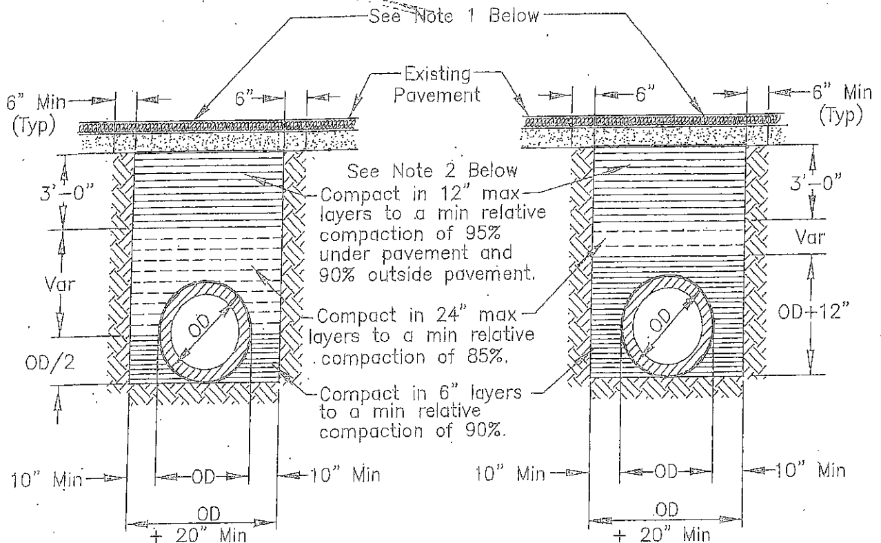
FLEXIBLE CONDUIT
