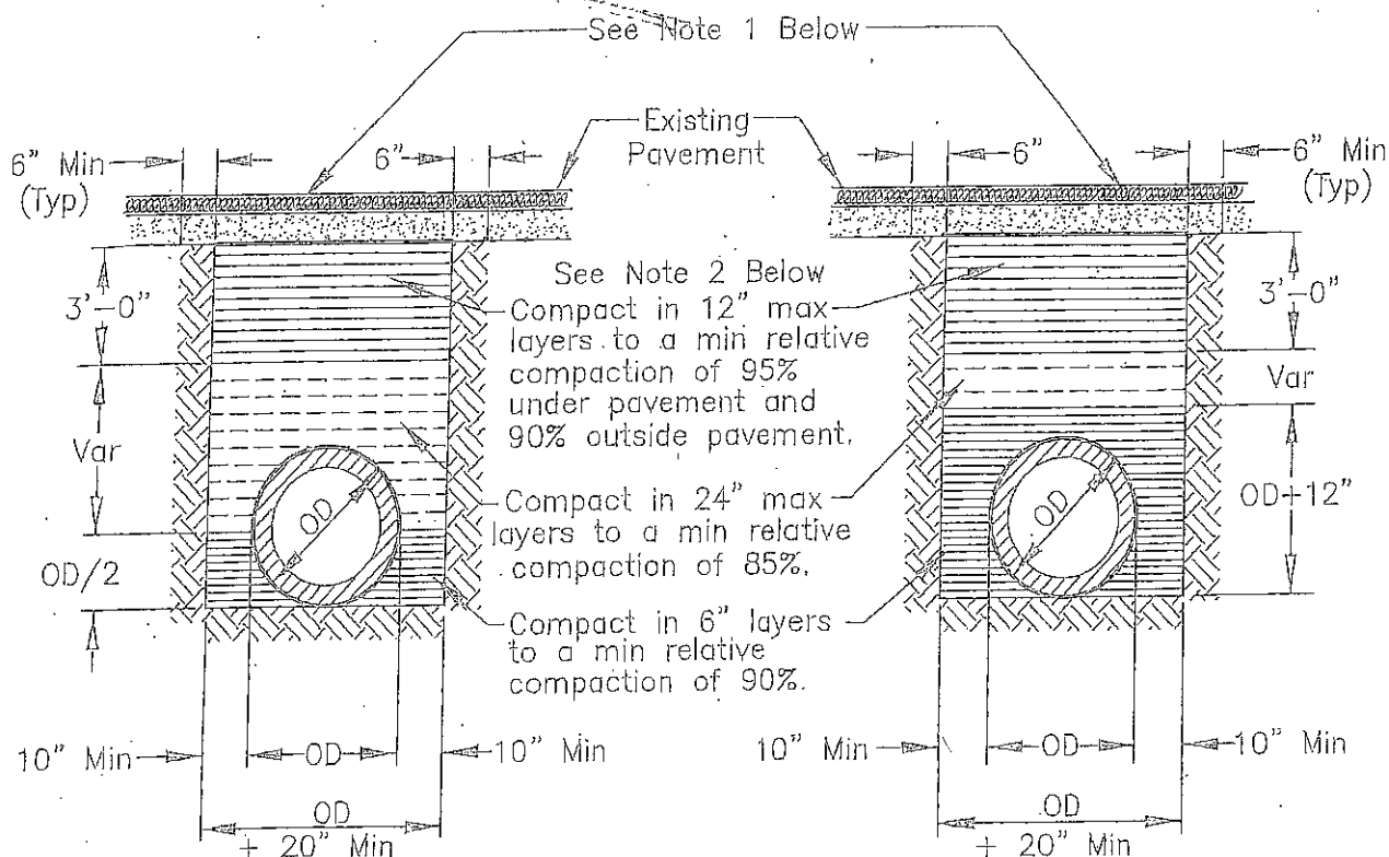
FLEXIBLE CONDUIT
