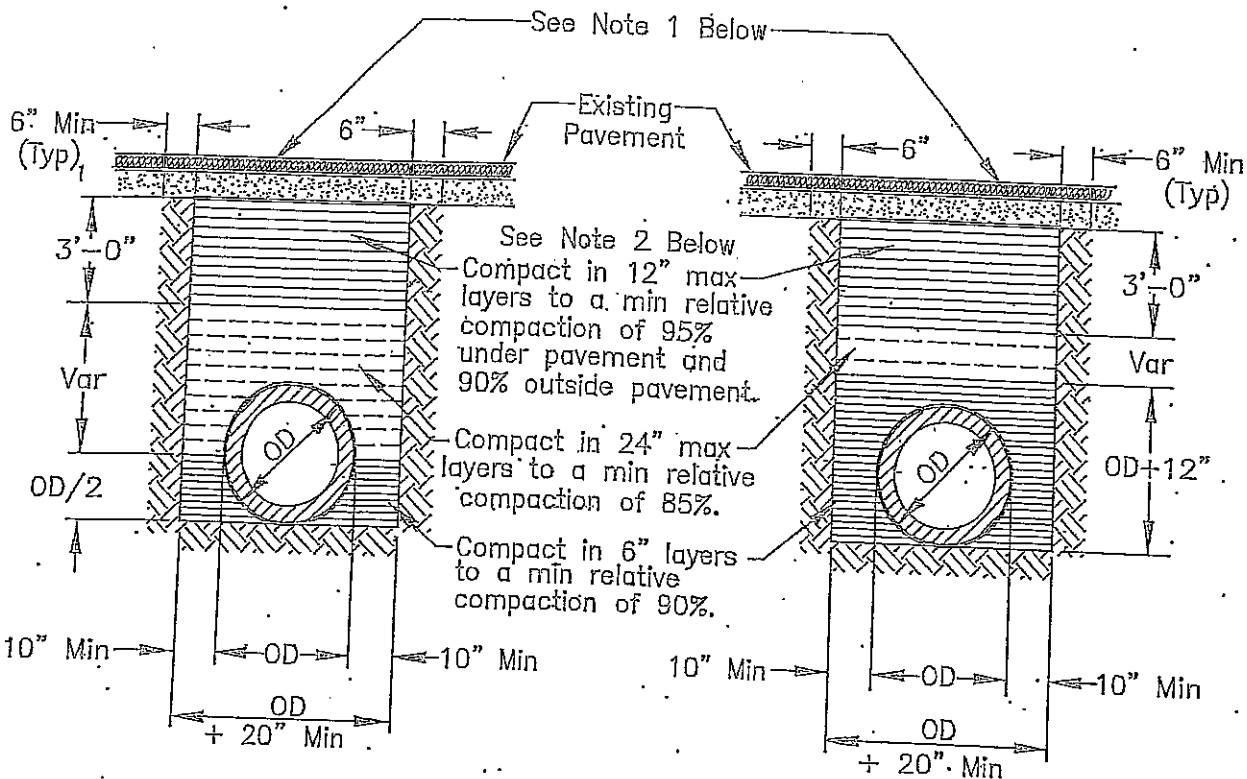
RIGID CONDUIT
