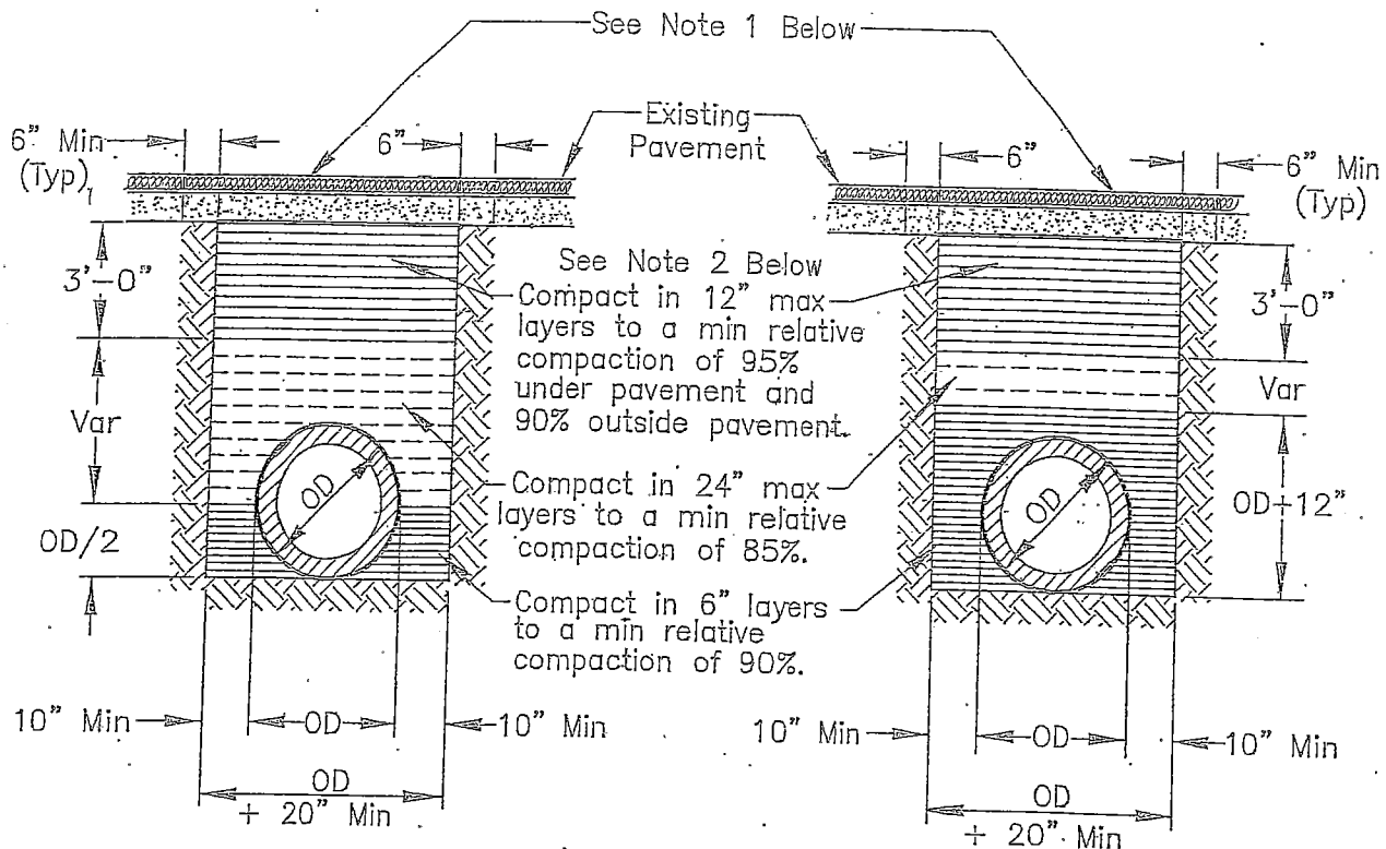
RIGID CONDUIT
