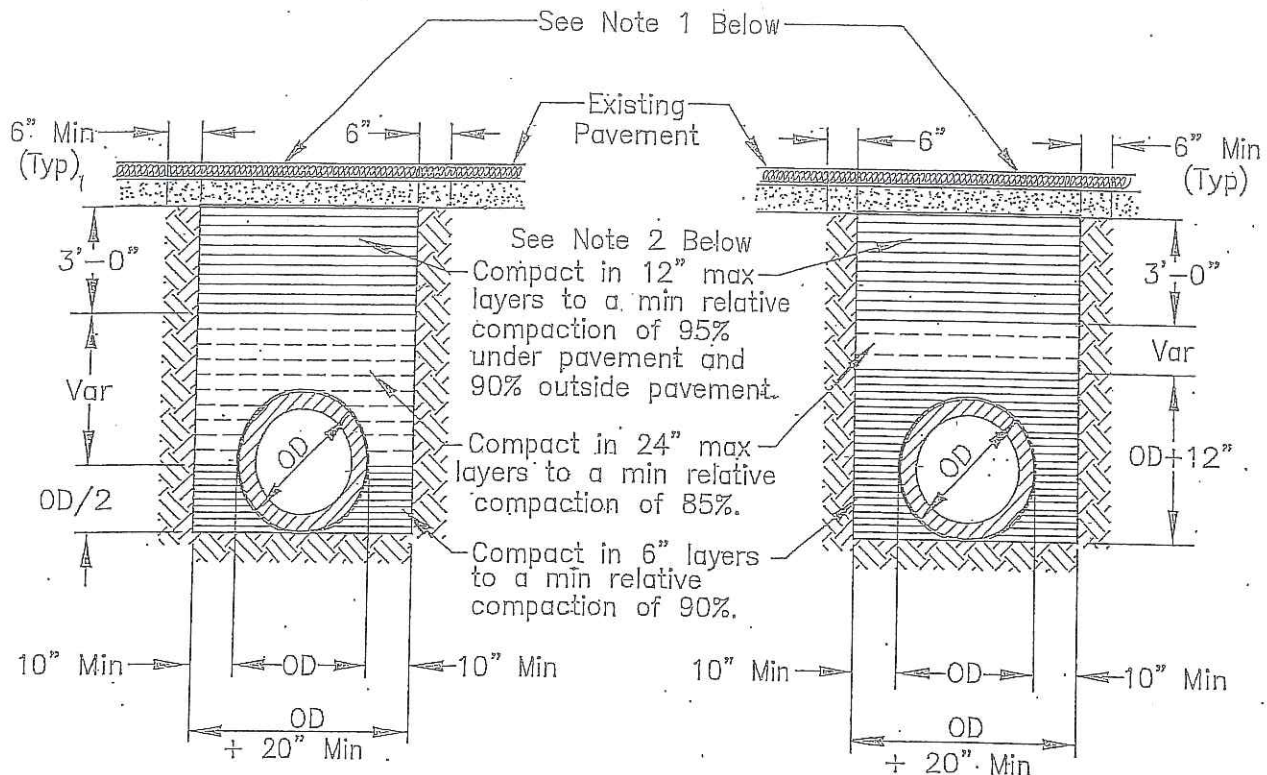
RIGID CONDUIT
