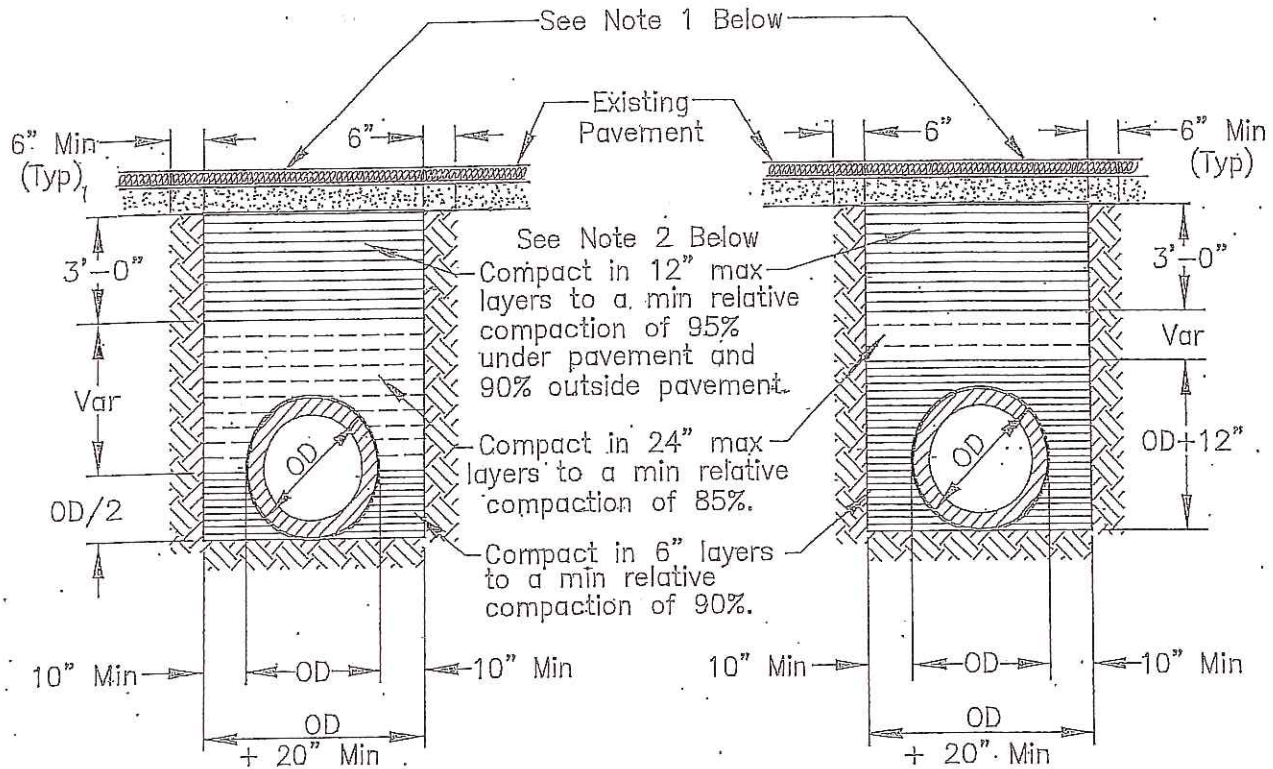
FLEXIBLE CONDUIT
