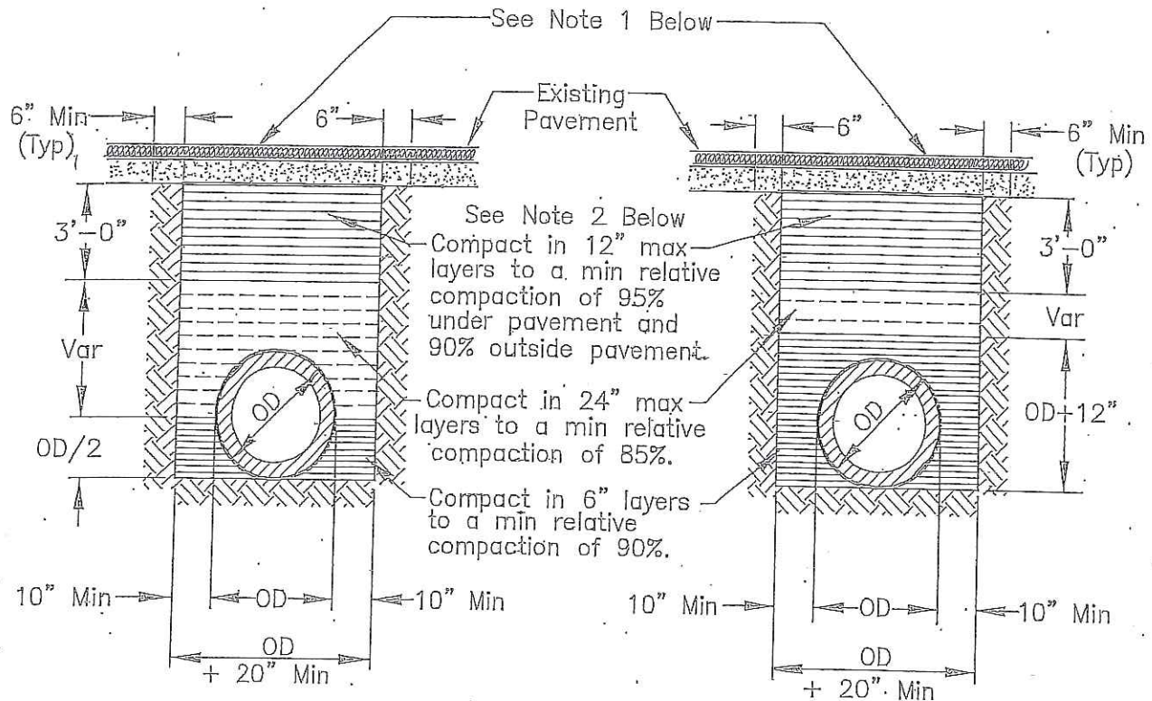
RIGID CONDUIT
