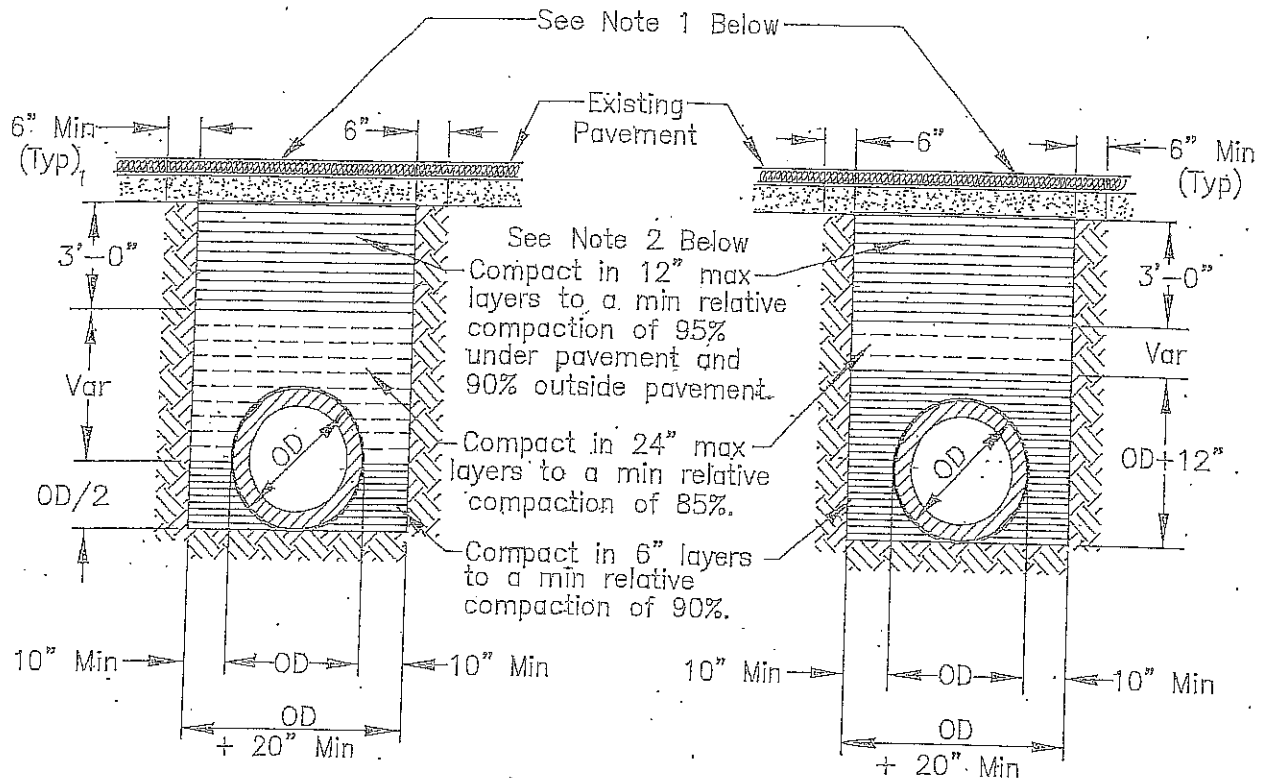
RIGID CONDUIT
