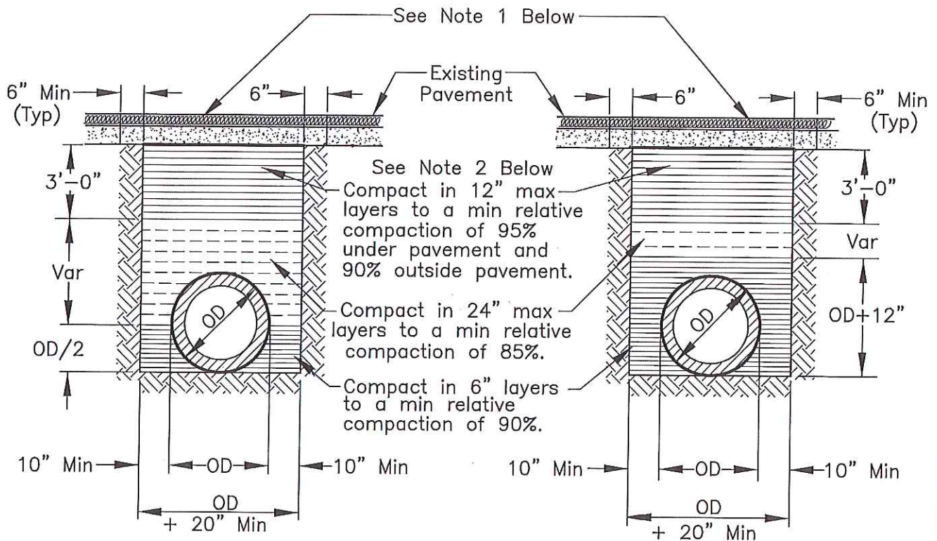
RIGID CONDUIT
