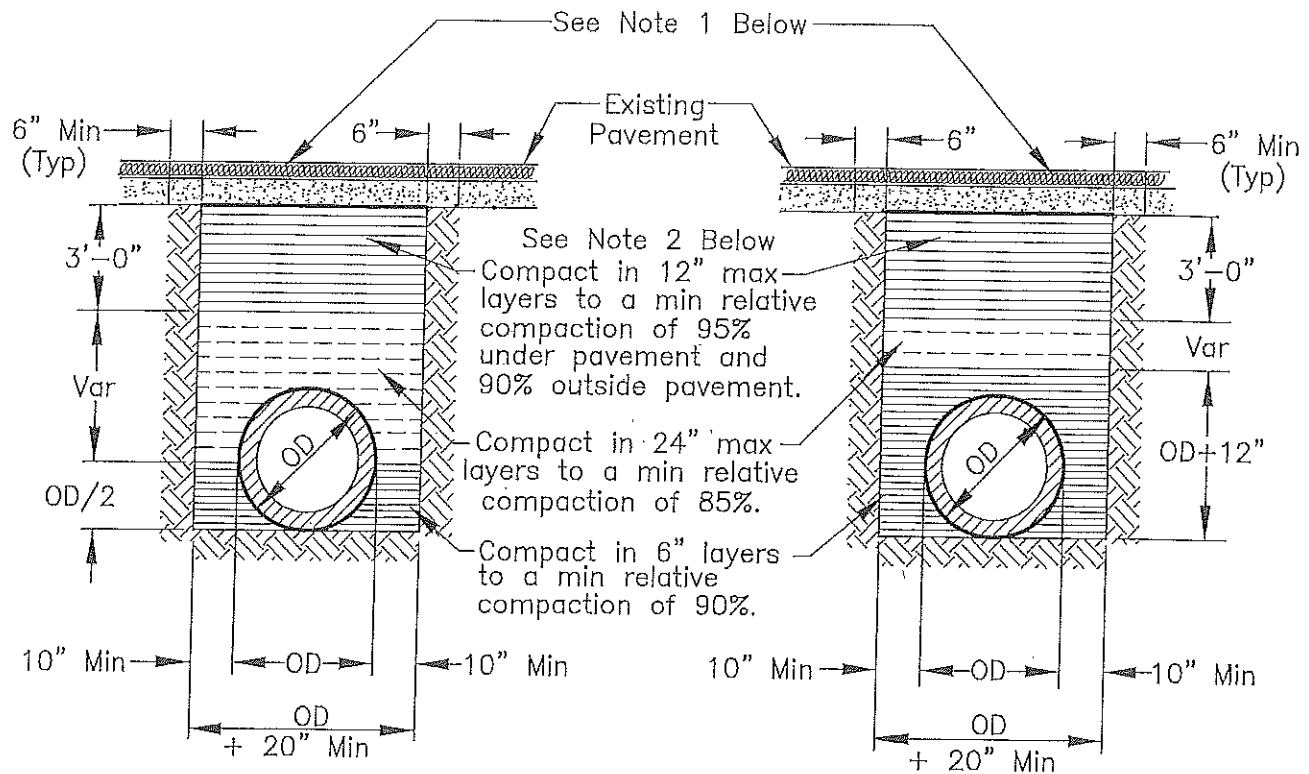
RIGID CONDUIT
