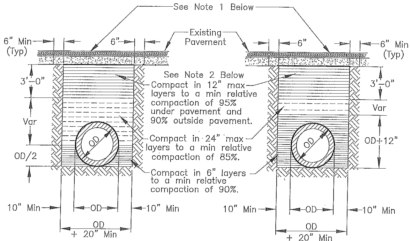
RIGID CONDUIT
