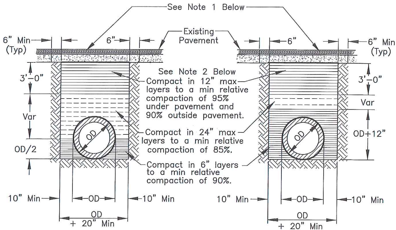
RIGID CONDUIT
