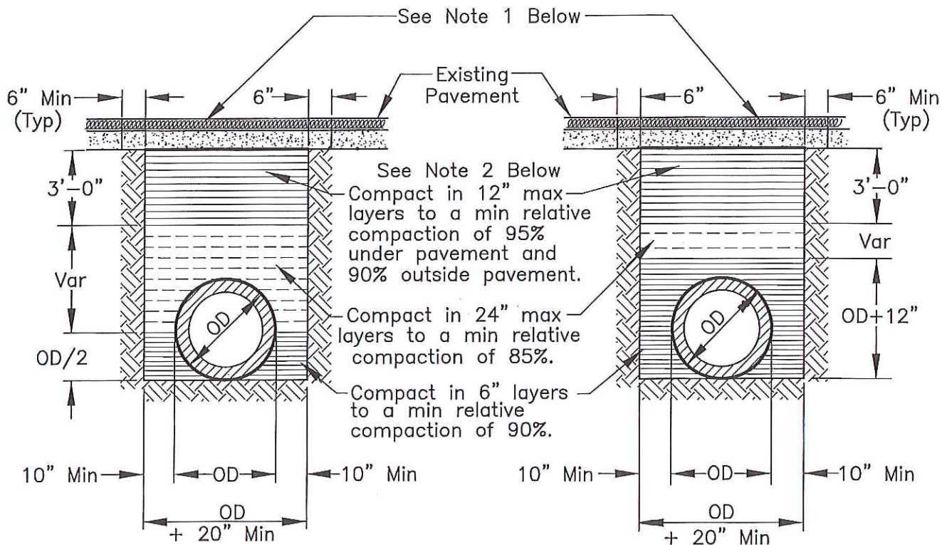
RIGID CONDUIT
