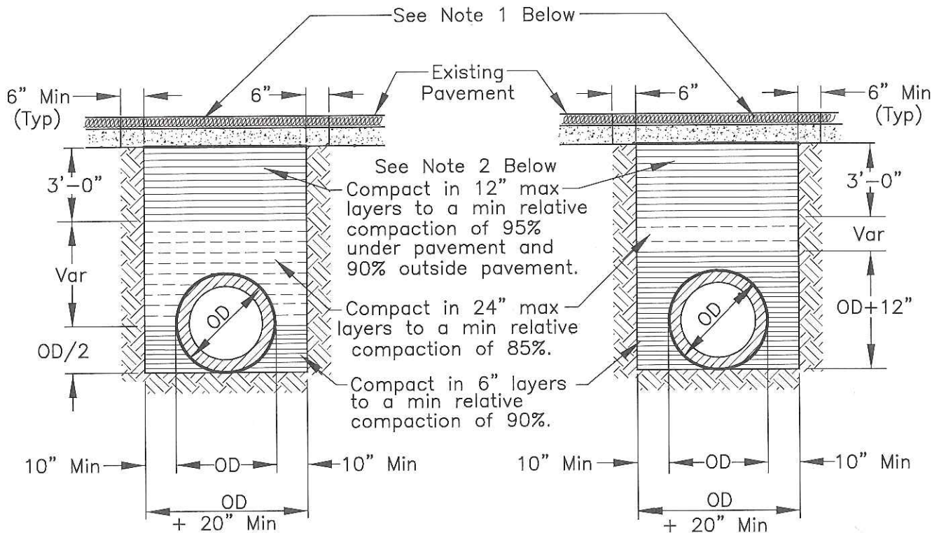
FLEXIBLE CONDUIT
