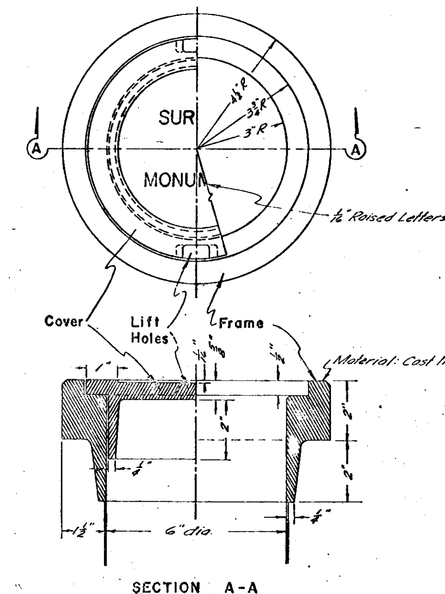
SECTION A-A
