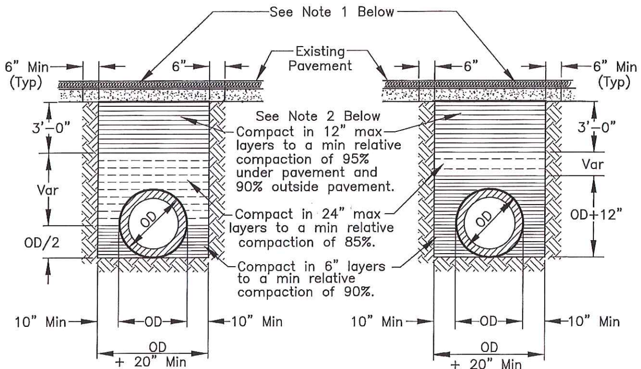
RIGID CONDUIT
