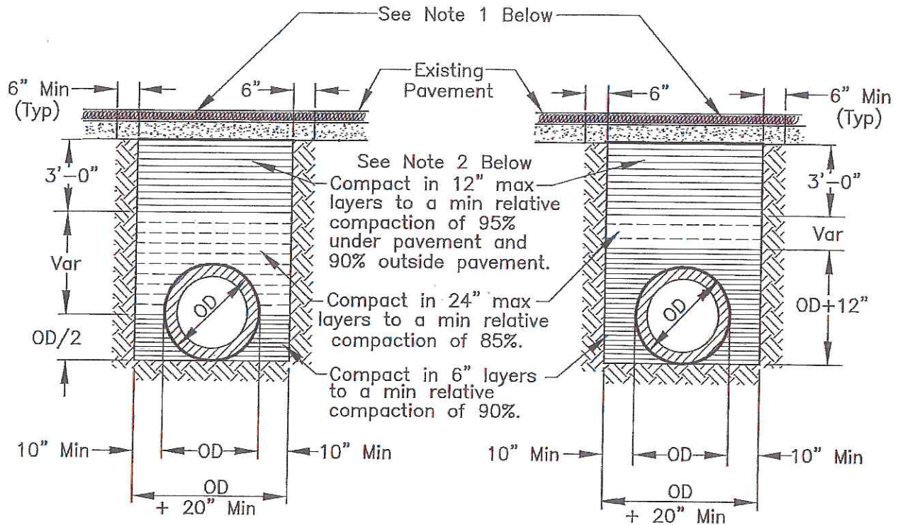
RIGID CONDUIT
