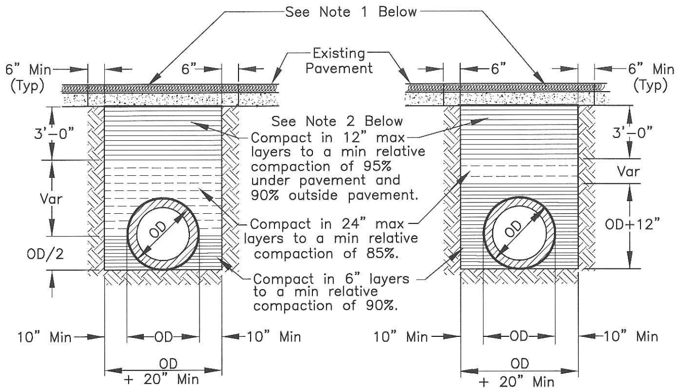
RIGID CONDUIT
