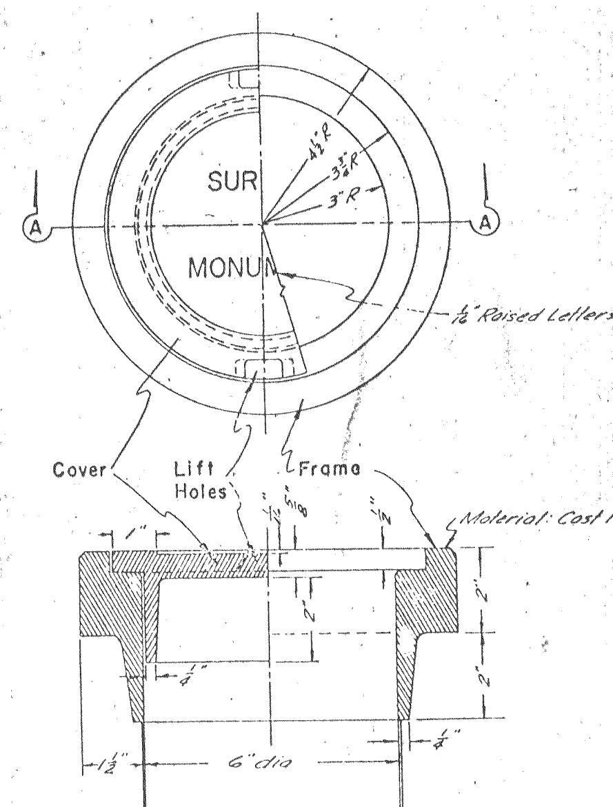
SECTION A-A
