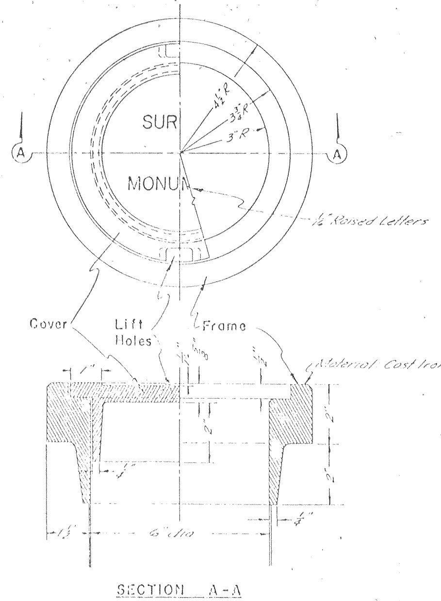
SECTION A-A
