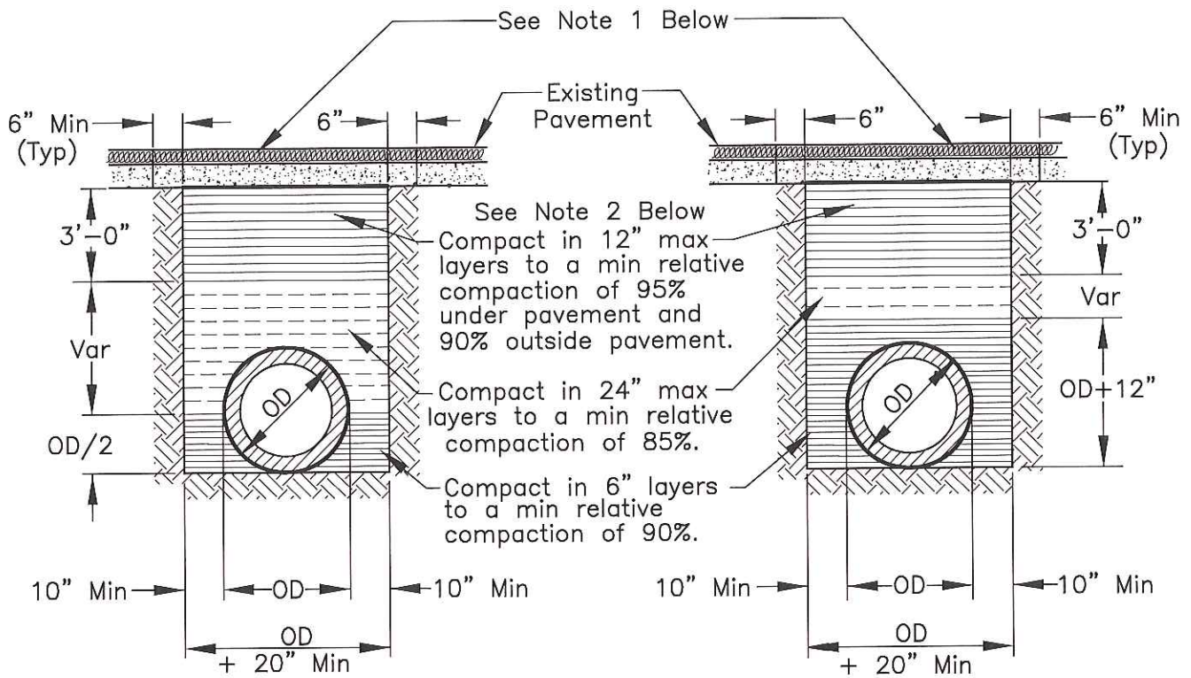
FLEXIBLE CONDUIT
